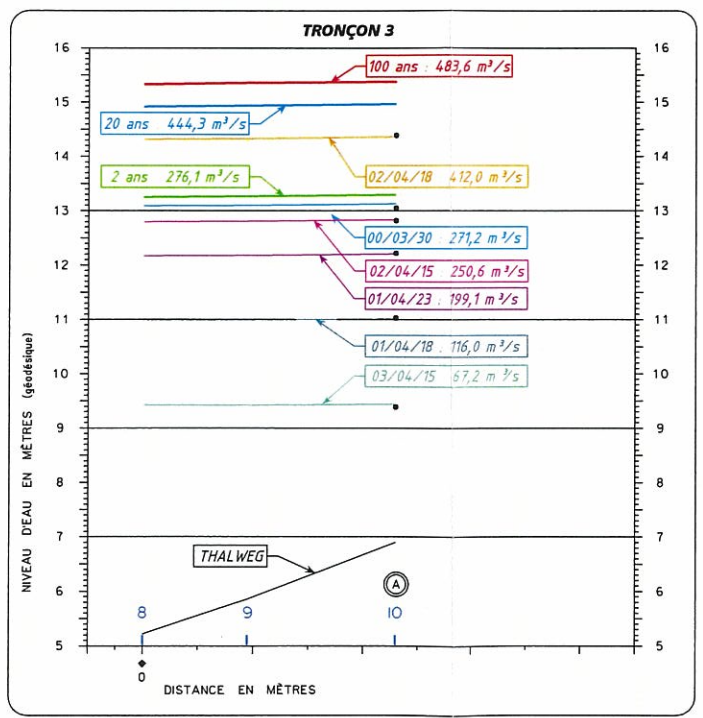
FIGURE 4 PROFIL DES PLANS D'EAU DES RIVIÈRES L'ASSOMPTION ET OUAREAU
