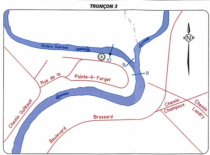
FIGURE 3 VUE EN PLAN DES RIVIÈRES L'ASSOMPTION ET OUAREAU ET LOCALISATION DES SECTIONS TRANSVERSALES ET DES SITES D'OBSERVATION DE NIVEAUX D'EAU
